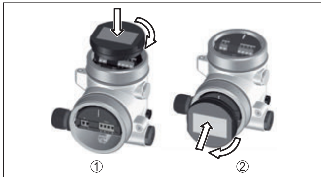
Рис. 8: Установка модуля индикации и настройки в двухкамерном корпусе
