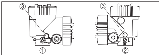
Рис. 2: Позиция фильтрующего элемента
