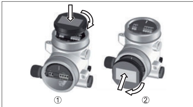
Рис. 8: Установка модуля индикации и настройки в двухкамерном корпусе 1 В отсеке электроники 2 В отсеке подключения
