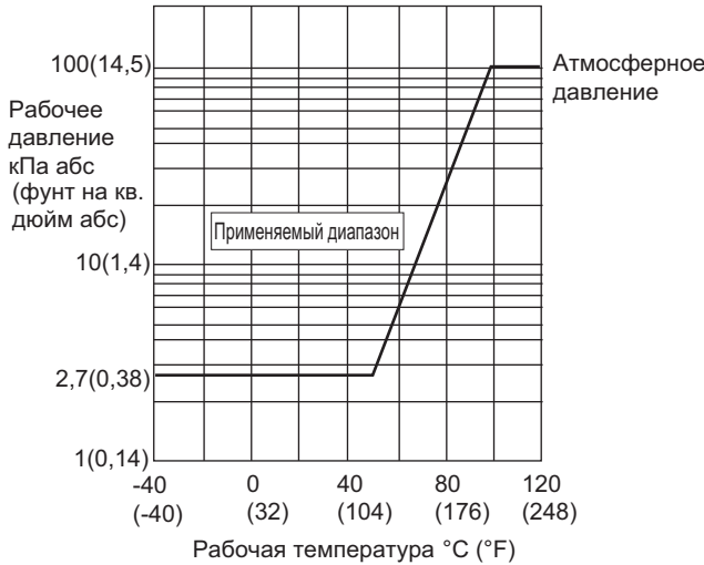
Рис. 1. Рабочее давление и рабочая температура
